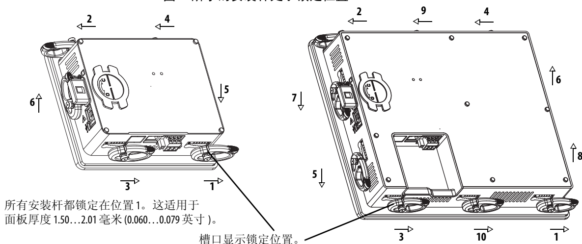
图 2- 所示的安装杆处于锁定位置
